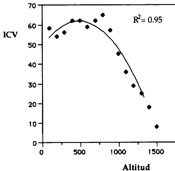
Fig. 2.- Relación entre el índice de complejidad de la vegetación (ICV) y la altitud, realizado a partir de los muestreos. [Relationship between the index of vegetation complexity (ICV) and altitude, made from census data.]
